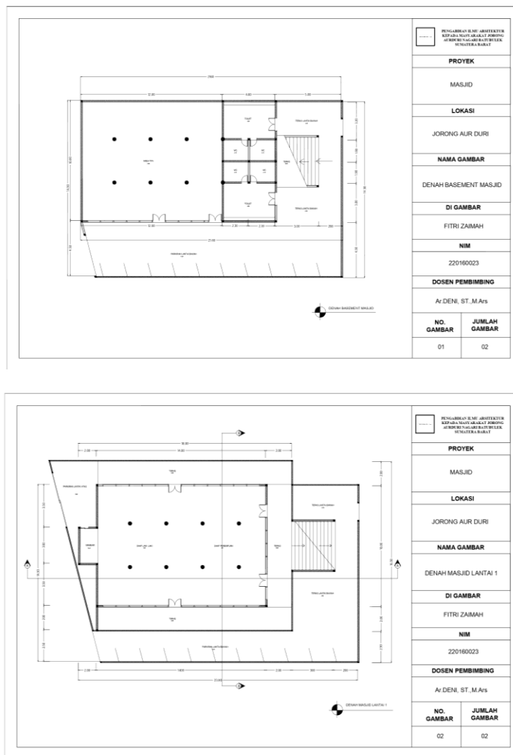
Gambar 2. Denah Masjid Basement dan Lantai 1
